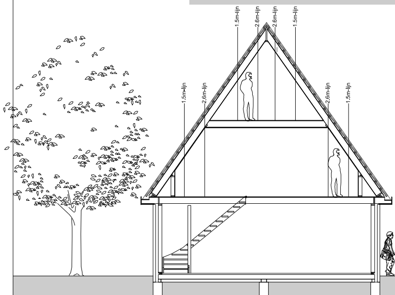
DOORSNEDE
